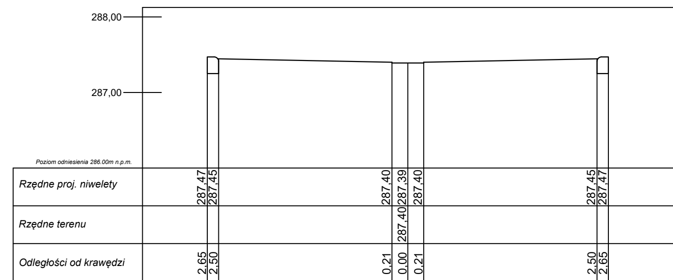
Przekrój poprzeczny odcinka nr III w km 0+036
