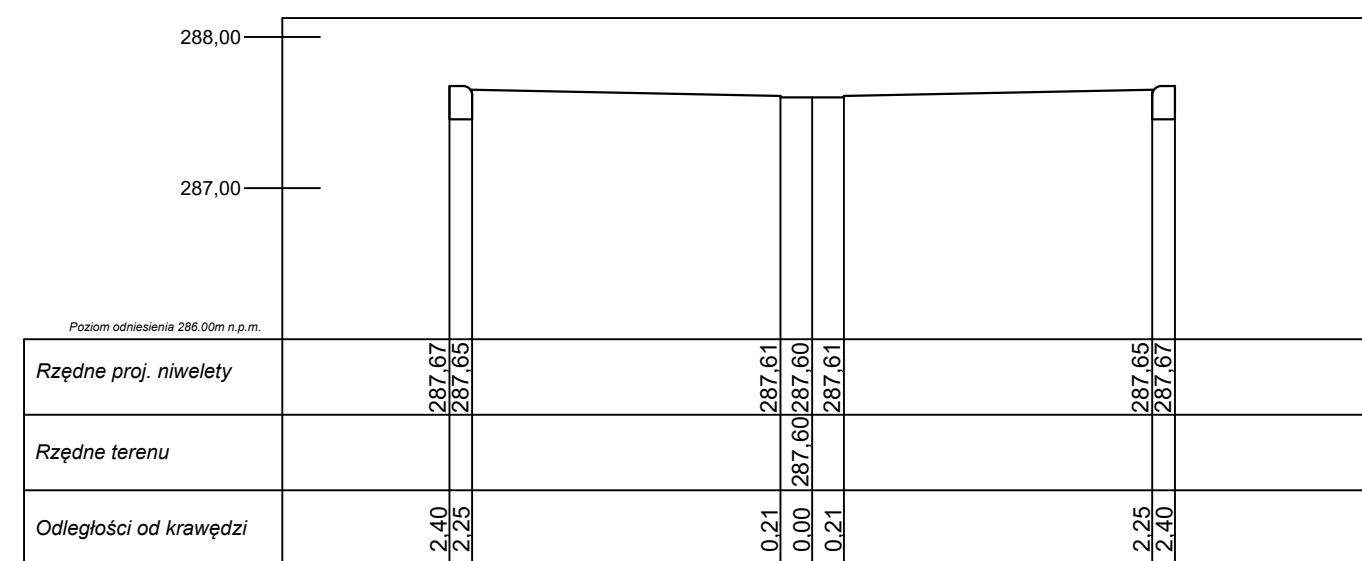
Przekrój poprzeczny odcinka nr II w km 0+027,76
