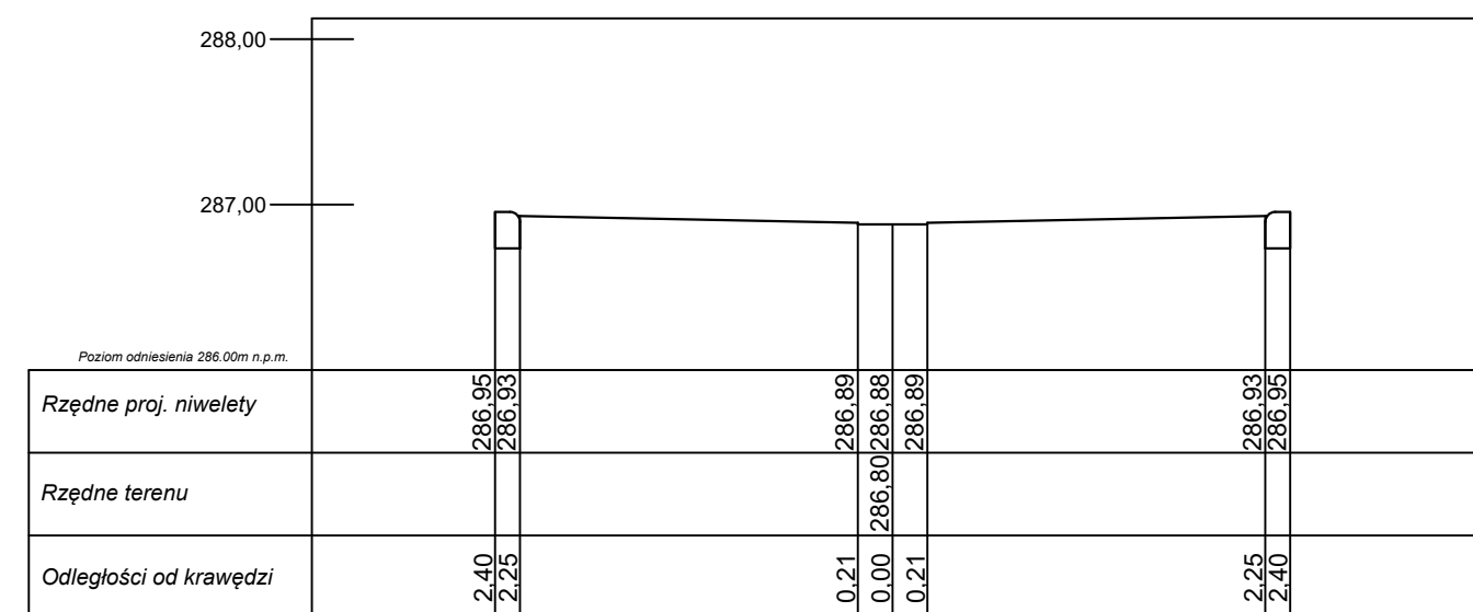
Przekrój poprzeczny odcinka nr IV w km 0+018,55
