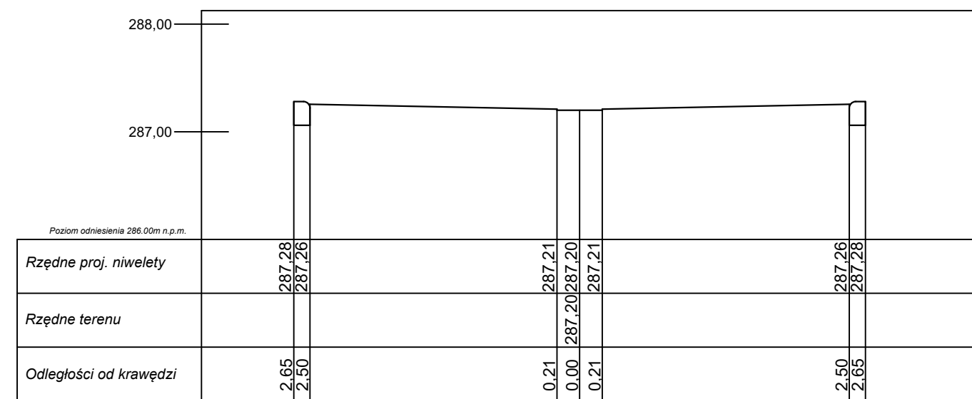
Przekrój poprzeczny odcinka nr I w km 0+043,3
