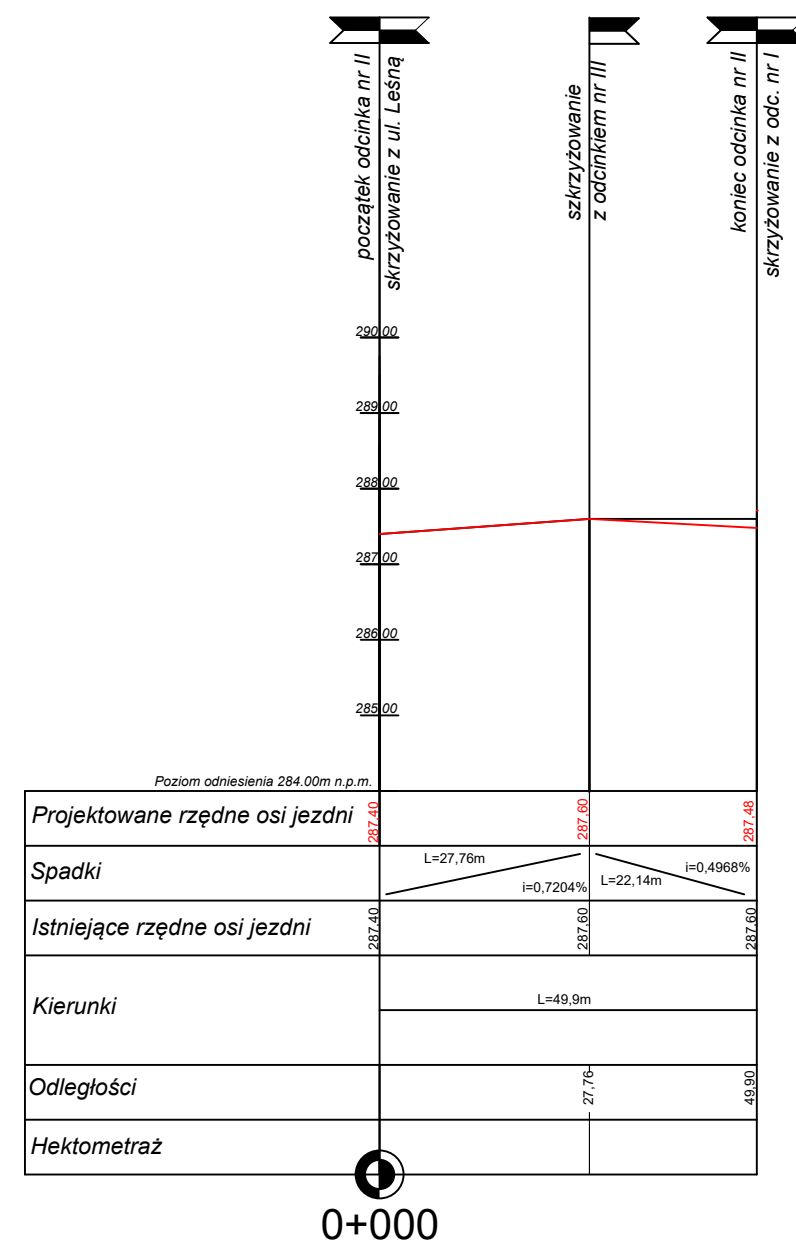
PROFIL PODŁUŻNY ODCINKA NR II
