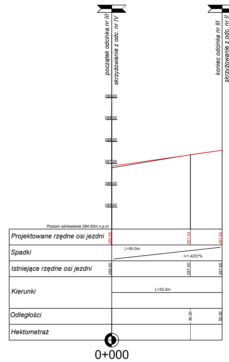
PROFIL PODŁUŻNY ODCINKA NR III
