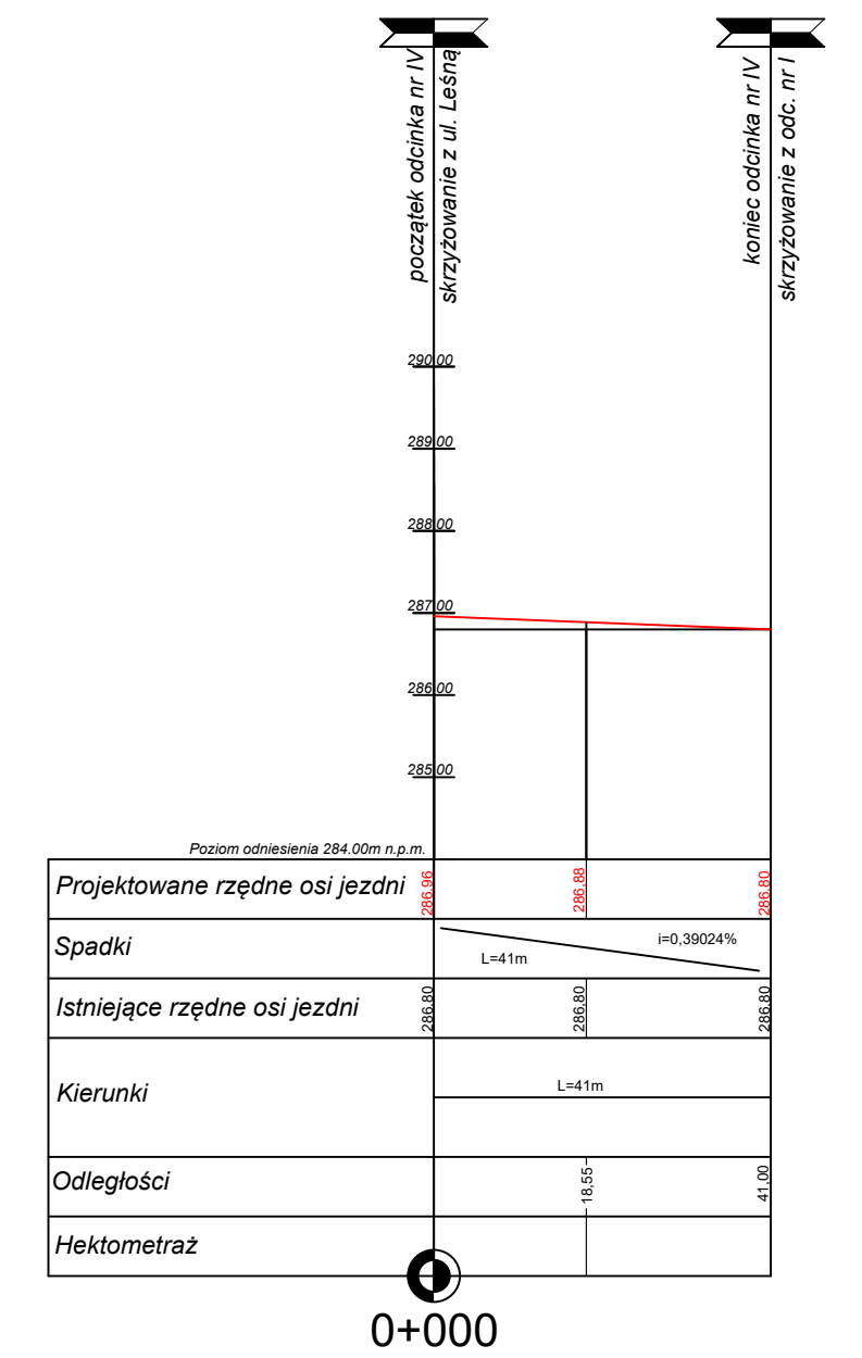
PROFIL PODŁUŻNY ODCINKA NR IV
