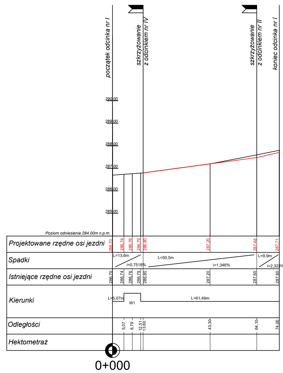
PROFIL PODŁUŻNY ODCINKA NR I
